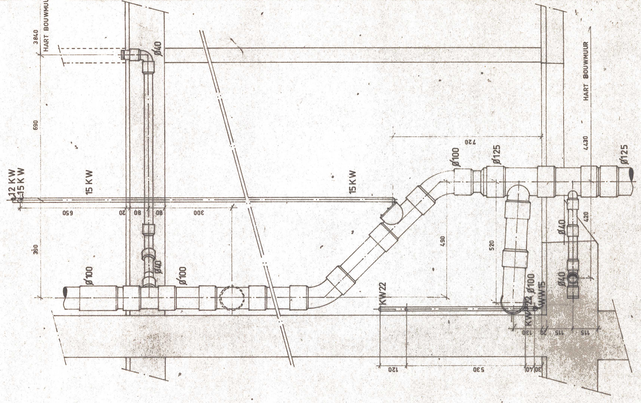
DOORSNEDE B-B
